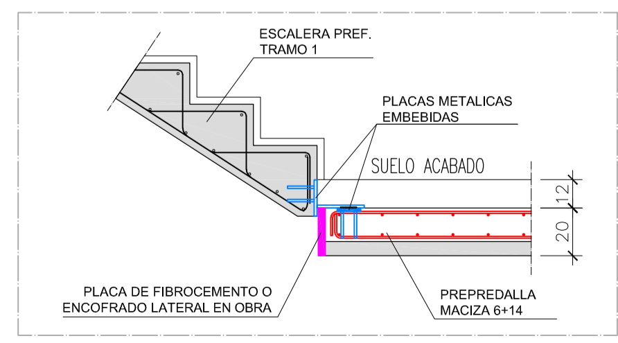
DETALLE E.1
