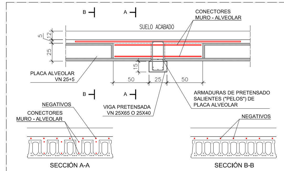
DETALLE 9 (ALZADO): APOYO DE PLACA ALVEOLAR SOBRE VIGA PRETENSADA VN 25x65 O 25x40
