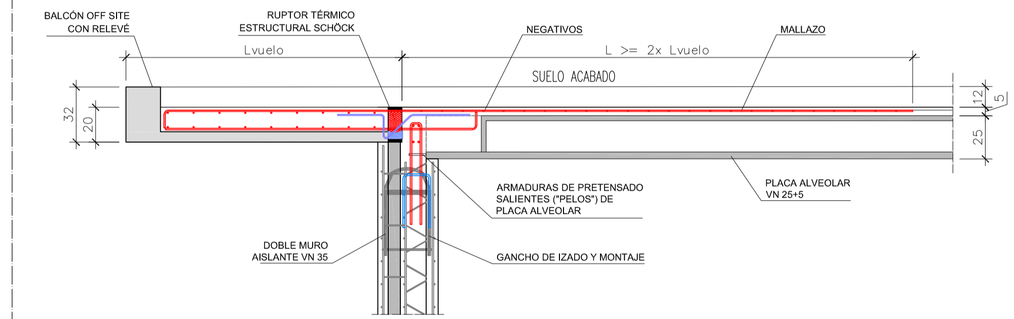
DETALLE 6 (ALZADO): CONEXIÓN DE BALCÓN OFF SITE A DOBLE MURO CON AISLANTE
