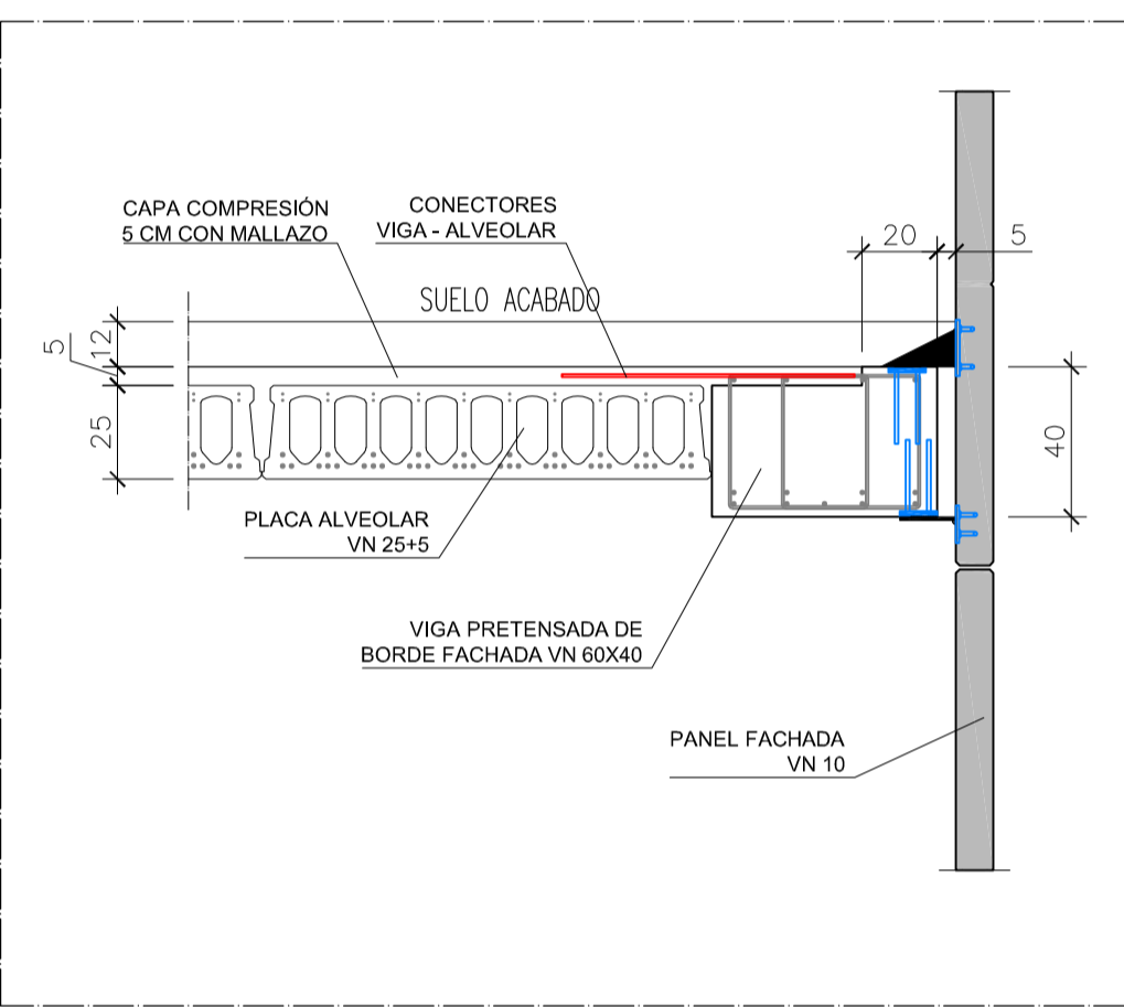
DETALLE 1 (ALZADO): ENCUENTRO DE VIGA PRETENSADA DE BORDE CON PANEL DE FACHADA
