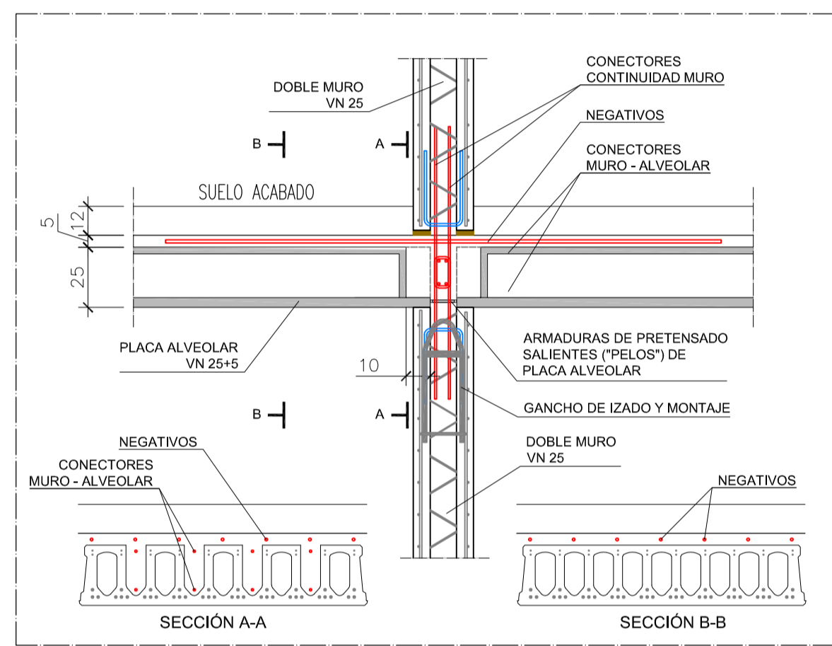
DETALLE 2 (ALZADO): APOYO DE PLACA ALVEOLAR SOBRE DOBLE MURO ESTRUCTURAL Y PROLONGACIÓN DE DOBLE MURO
