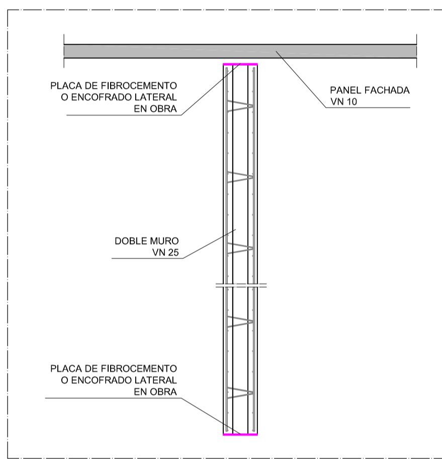
DETALLE 4 (PLANTA): UBICACIÓN DE PLACAS DE FIBROCEMENTO PARA EVITAR ENCOFRADOS LATERALES EN HUECOS GENERADOS EN DOBLE MURO PARA PUERTAS Y VENTANAS
