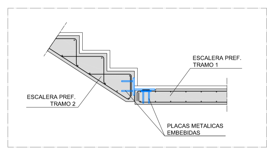
DETALLE E.3
