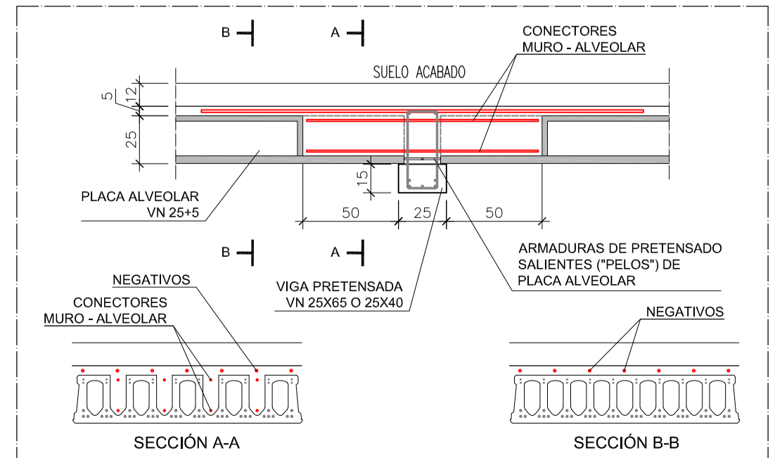
DETALLE 9 (ALZADO): APOYO DE PLACA ALVEOLAR SOBRE VIGA PRETENSADA VN 25x65 O 25x40
