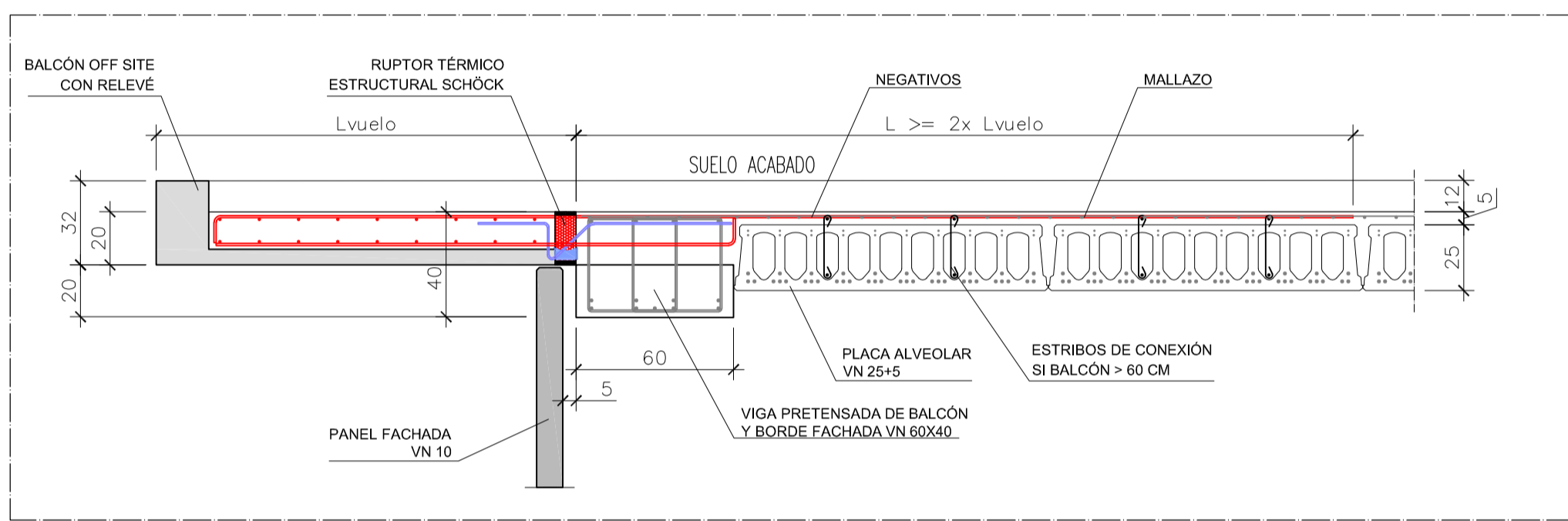
DETALLE 5 (ALZADO): CONEXIÓN DE BALCÓN OFF SITE A VIGA PRETENSADA DE BORDE DE FACHADA
