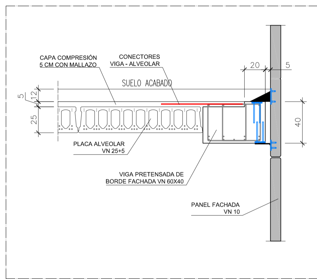
DETALLE 1 (ALZADO): ENCUENTRO DE VIGA PRETENSADA DE BORDE CON PANEL DE FACHADA
