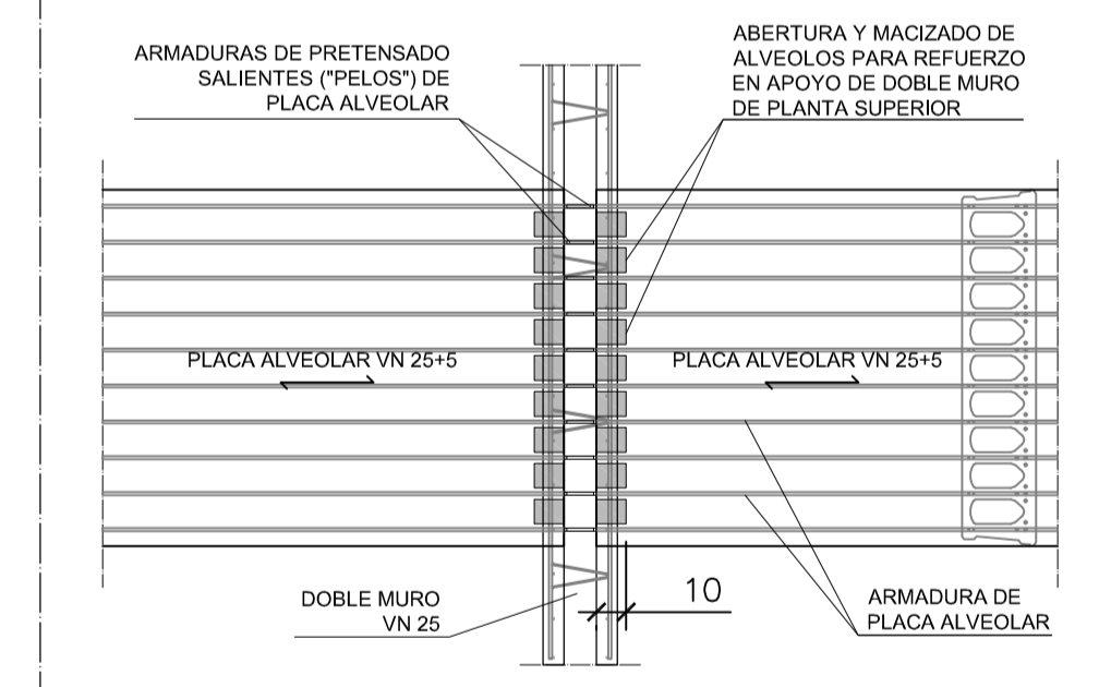
DETALLE 7 (PLANTA): APOYO DE PLACA ALVEOLAR SOBRE DOBLE MURO ESTRUCTURAL Y SOBRE VIGA PRETENSADA VN 25x45
