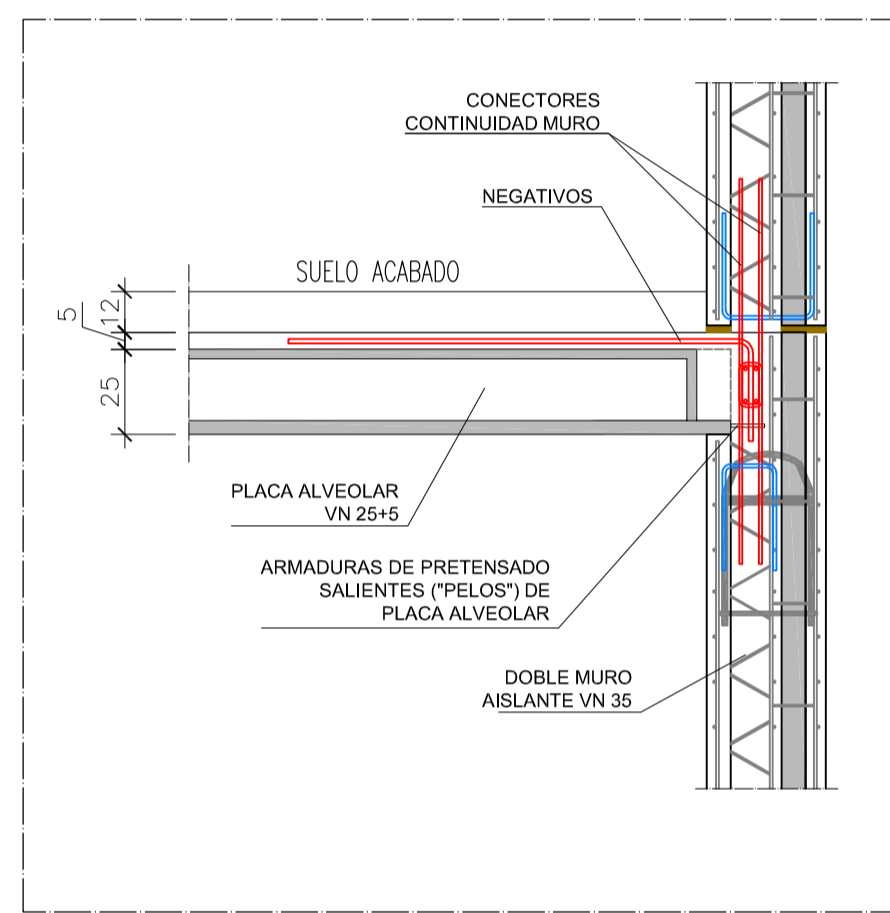
DETALLE 3 (ALZADO): APOYO DE PLACA ALVEOLAR SOBRE DOBLE MURO AISLANTE ESTRUCTURAL
