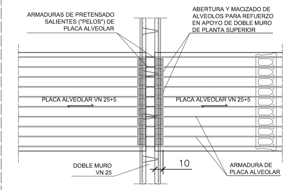
DETALLE 7 (PLANTA): APOYO DE PLACA ALVEOLAR SOBRE DOBLE MURO ESTRUCTURAL Y SOBRE VIGA PRETENSADA VN 25x45
