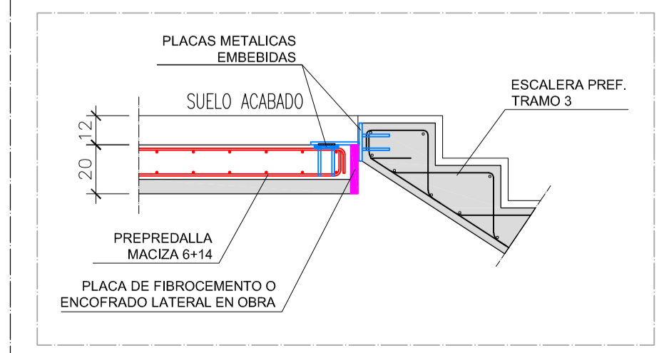
DETALLE E.6
