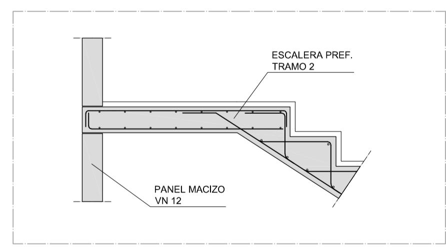
DETALLE E.2
